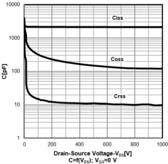
Typ. capacitances
