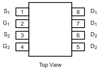
SO-8
