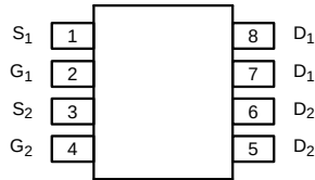
MSOP8
