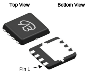
DFN 3x3
