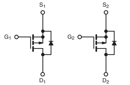
P-Channel MOSFET
